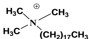
Octadecyltrimethylammonium (ODTMA)
